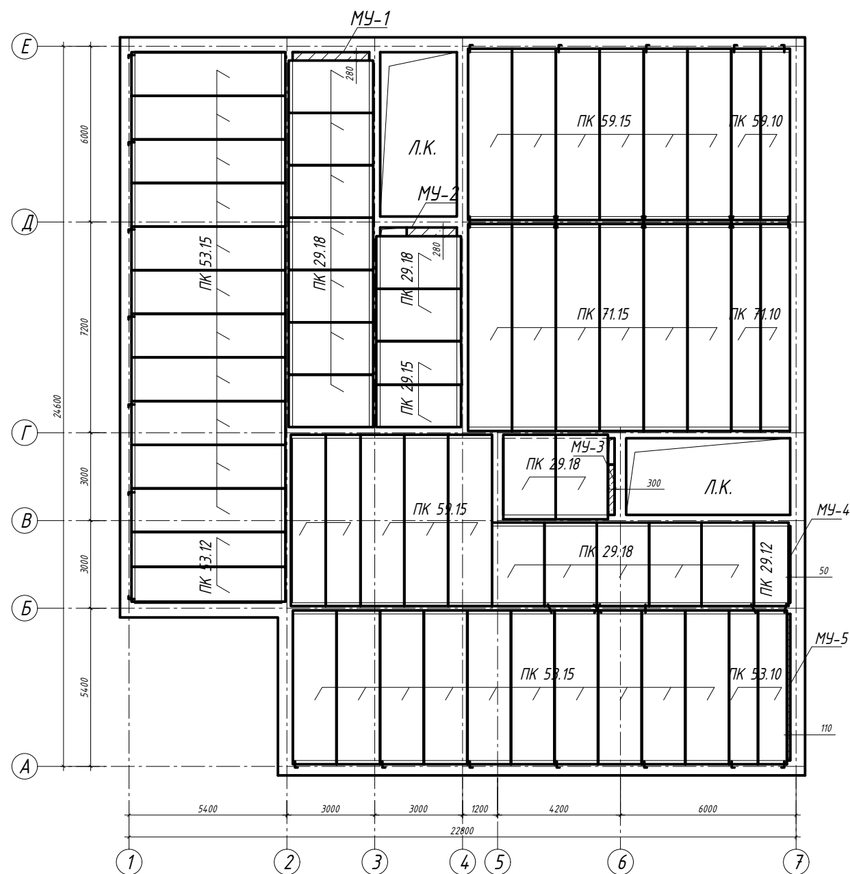
Схема расположения плит перекрытий на отм.+2,700
