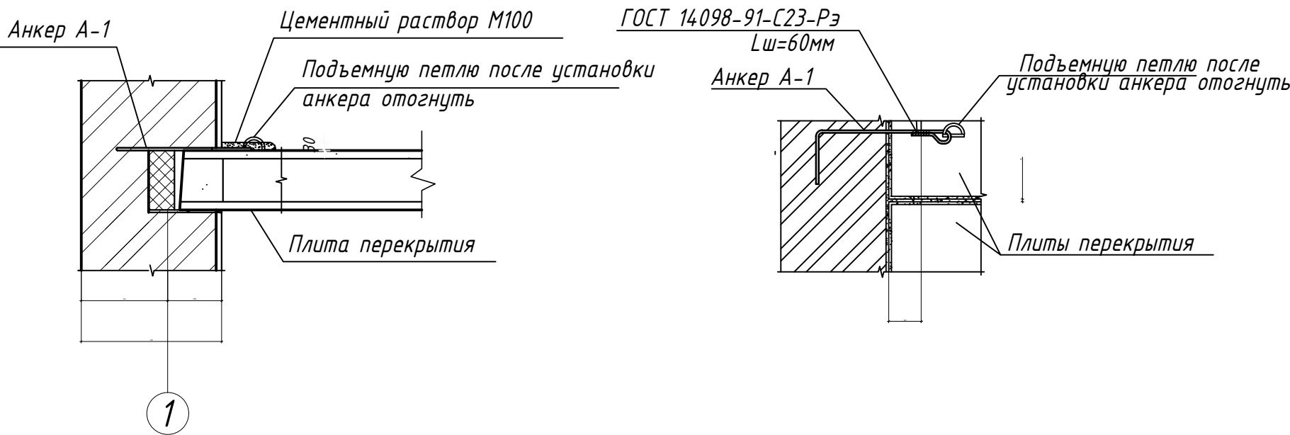
Узел опирания плиты перекрытия на наружную стену
